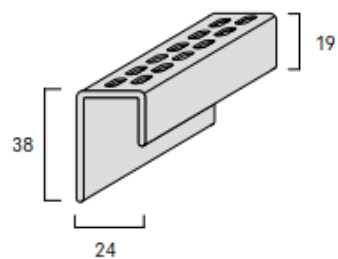
FS-261 U-планка универсальная (перфорированная)
