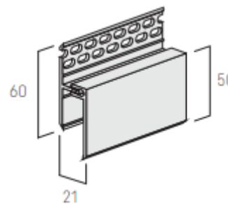
FS-262 Планка вентиляционная (двухкомпонентная)
