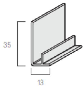
FS – 211 Планка стартовая
