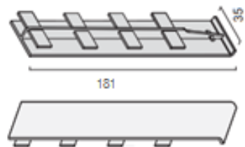
J-201 Соединитель для FS-201
