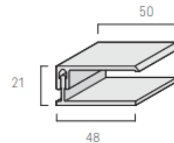
FS – 252 Финишная планка (двухкомпонентная)
